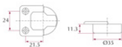
*Aplicación puertas abatibles
