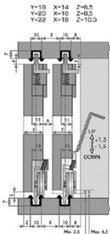
Detalle mecanizado y regulación.
