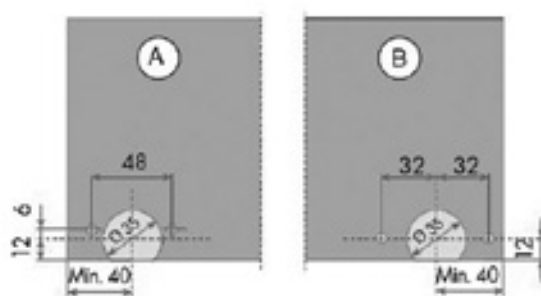
A - Mecanizado normal. B - Mecanizado sistema 32.
