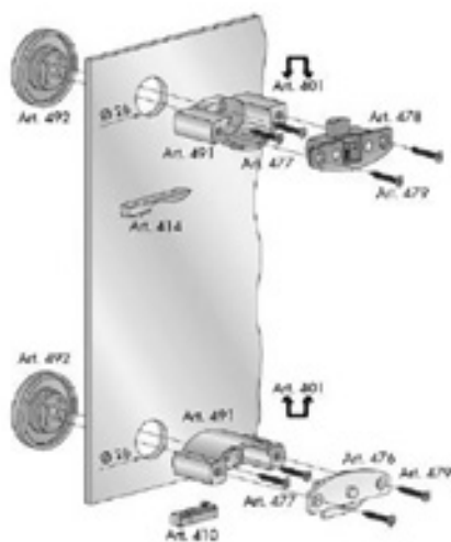
Esquema montaje.
