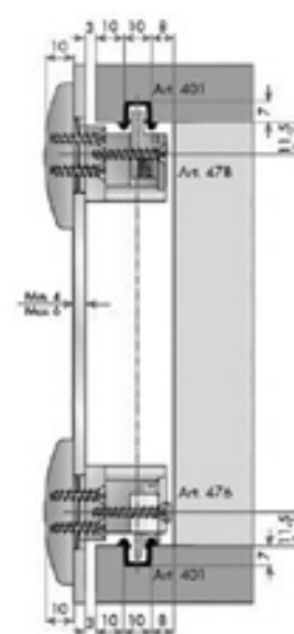
Aplicación interna puerta de cristal.
