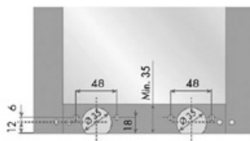
Mecanizado en puertas de cristal con marco de madera o aluminio.
