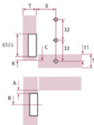
*Detalles mecanizado puerta cerrada
