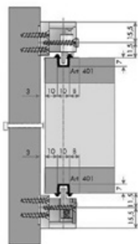
Aplicación externa puerta de madera.
