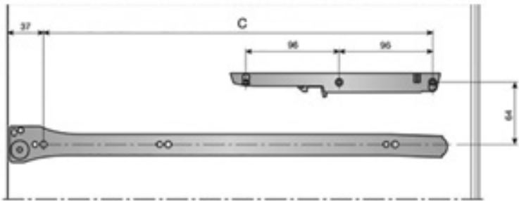
Fijación en el costado
