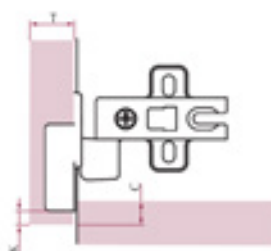
*Detalles mecanizado puerta cerrada
